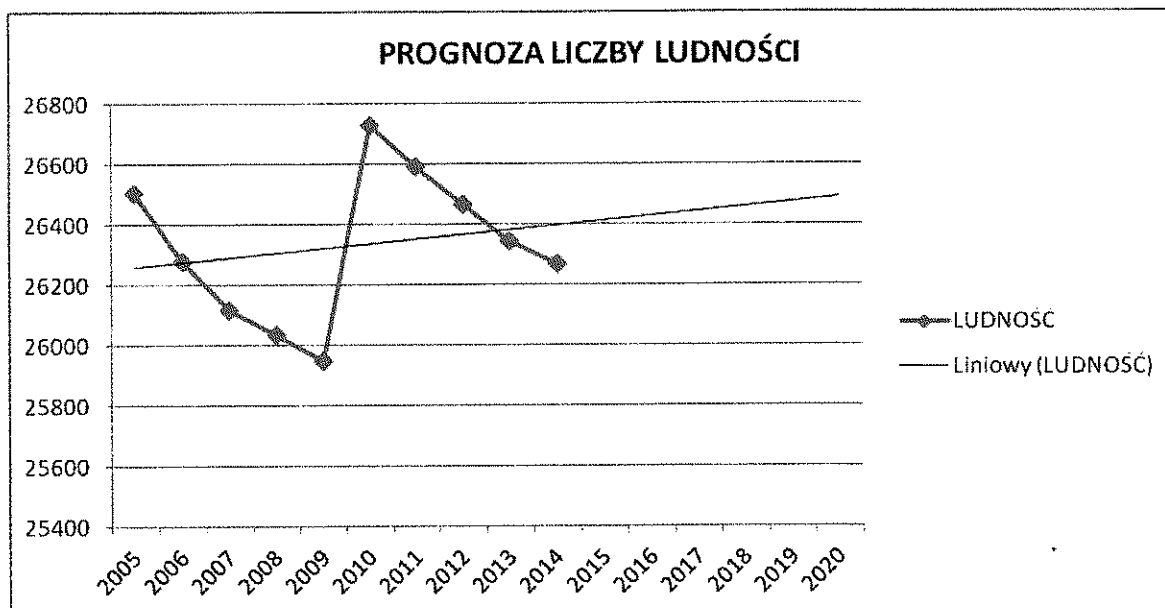
Wykres 3. Prognoza liczby ludności gminy Sokółka
